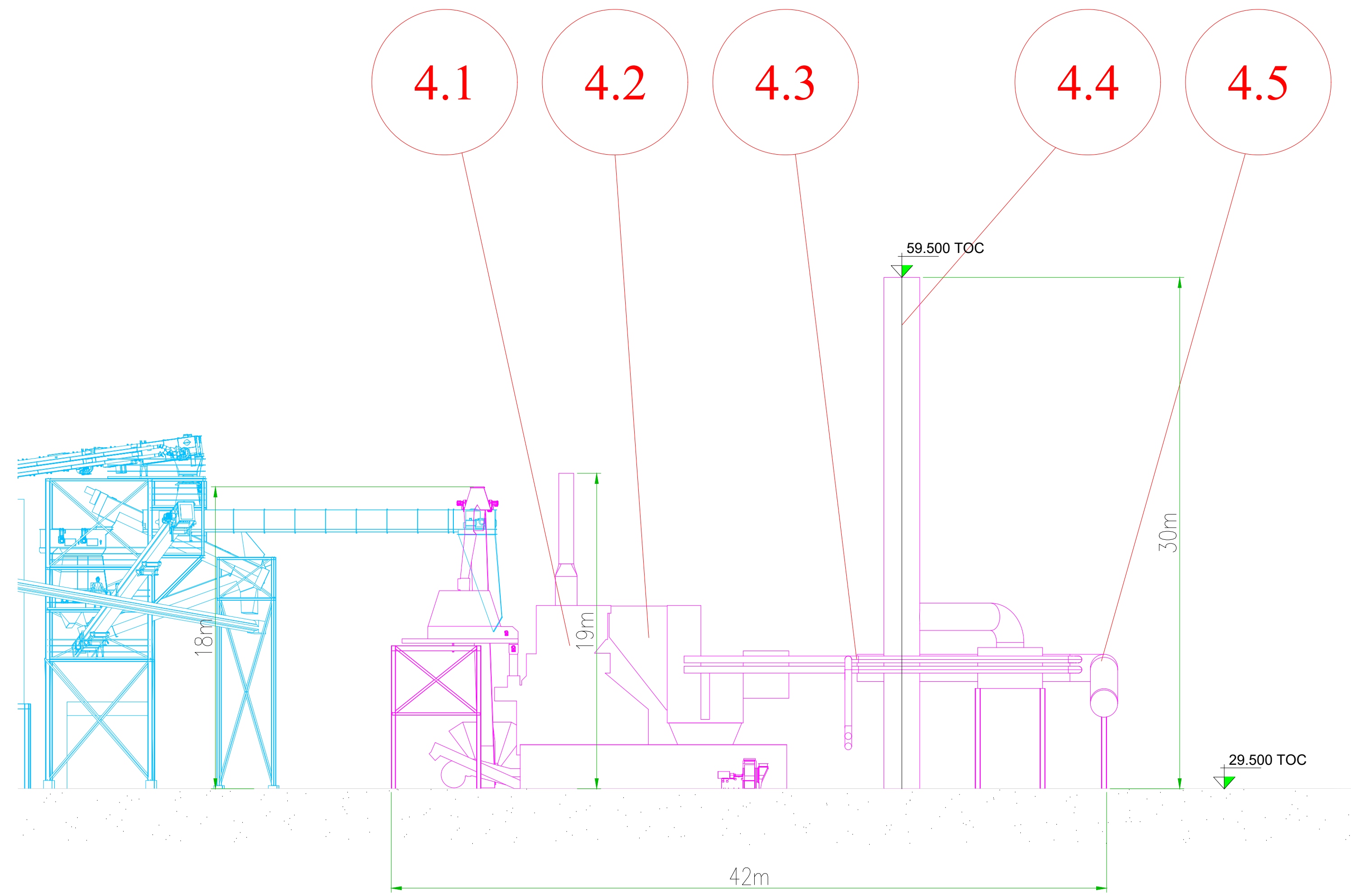
Section A-A
