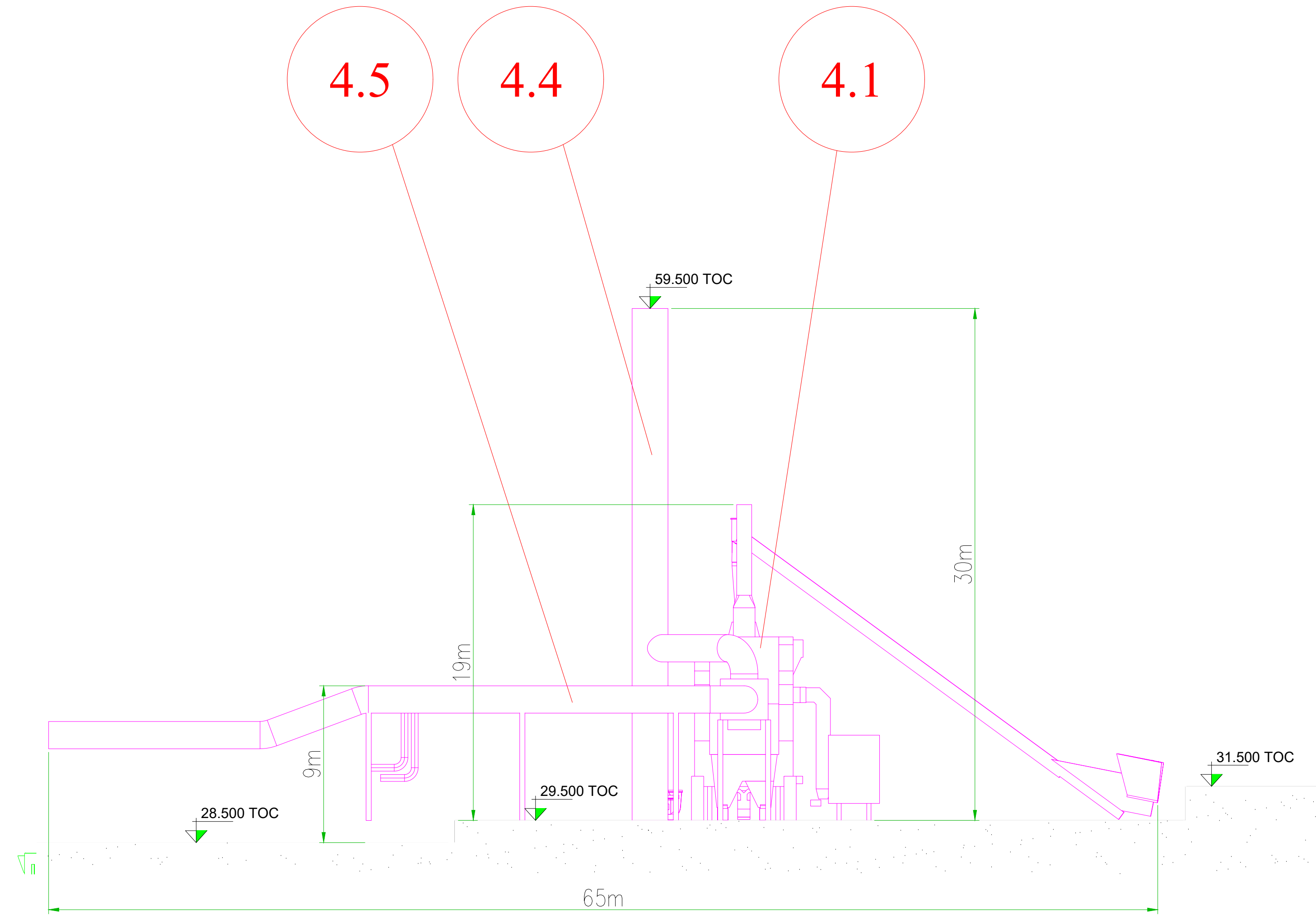
Section D-D
